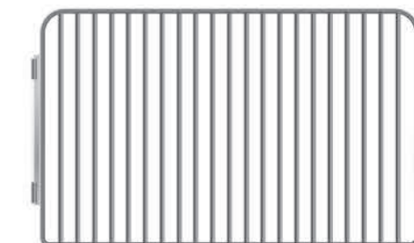
品番 HS-1500 1500 門 横幅1580mm(耳40mm左右)× 高さ930mm 【材質】鉄亜鉛メッキ 【発注単位】1枚
